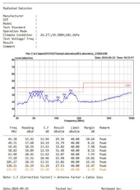
图 5-7 辐射测试垂直方向
