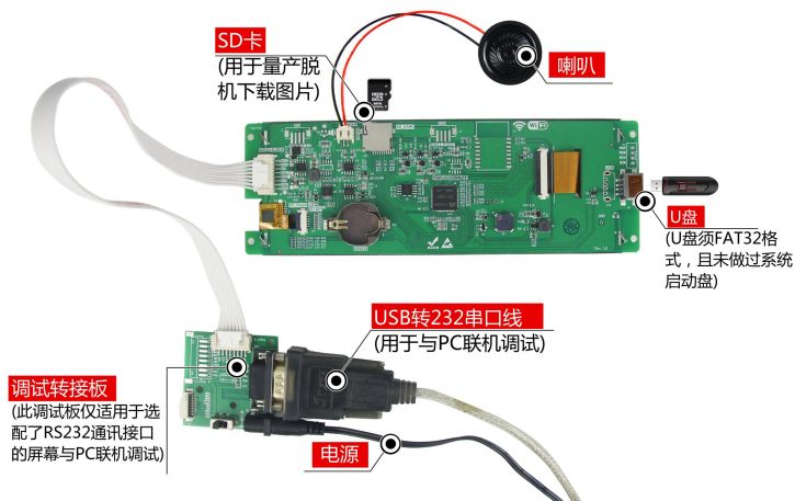
图 1-3 RS232 调试工具图
